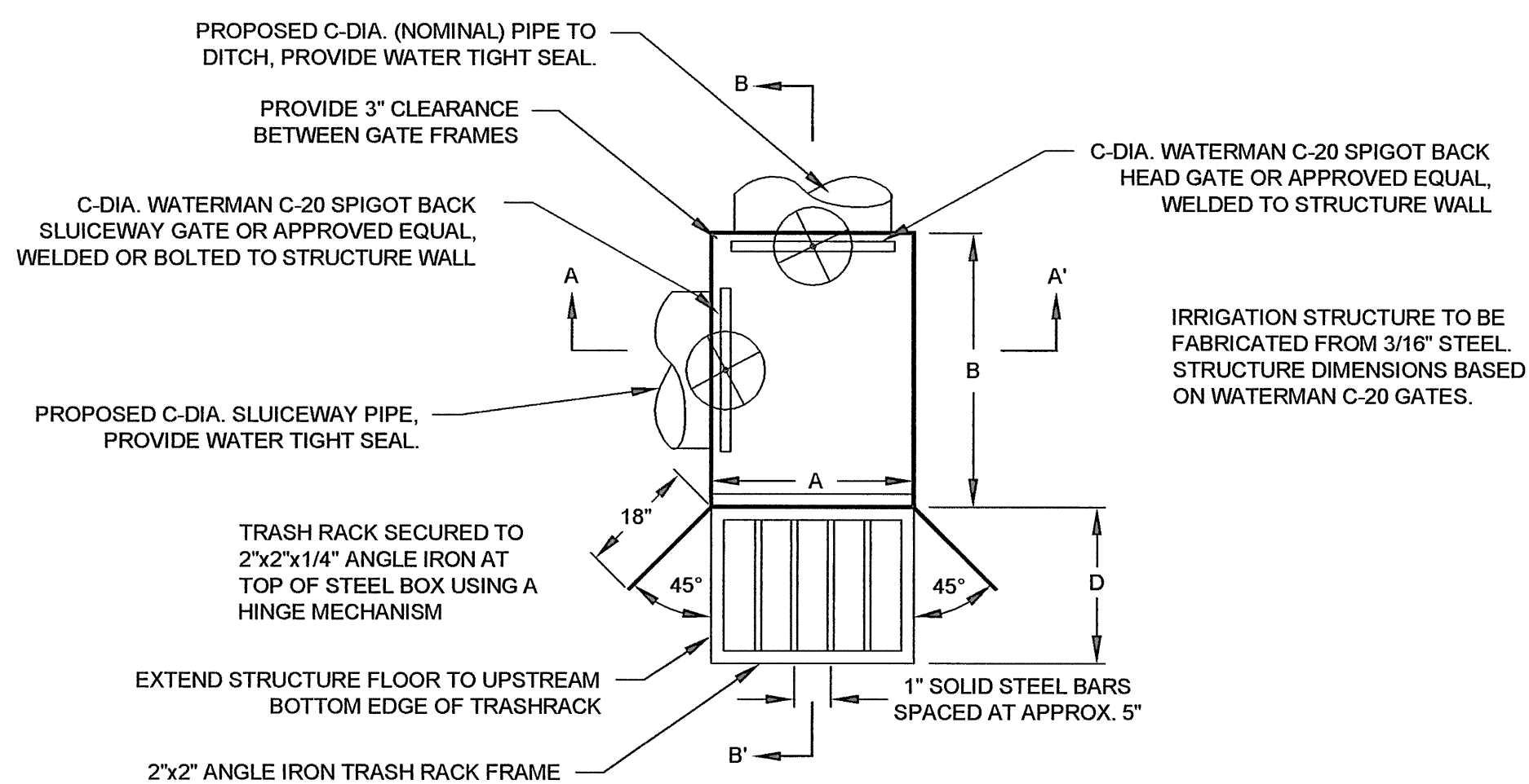
DETAIL: IRRIGATION HEADING STRUCTURE (N.T.S.)
