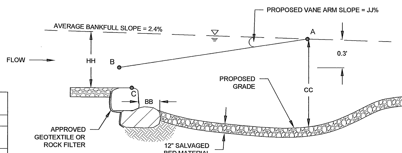
XS4 (N.T.S.)
