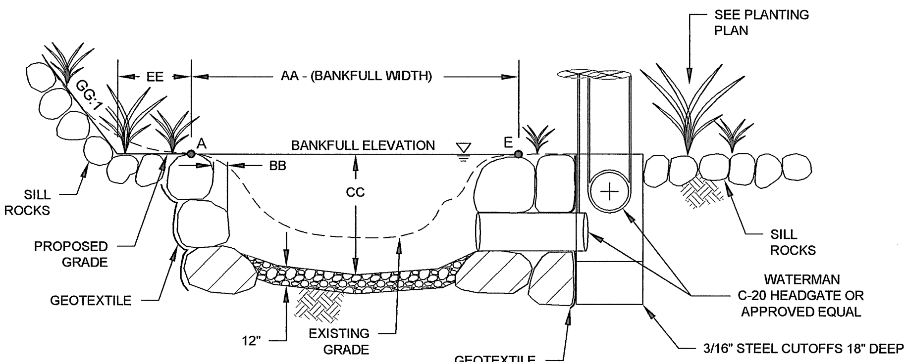
XS1 (N.T.S.)
