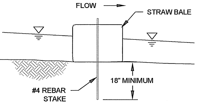
SECTION (N.T.S.)
