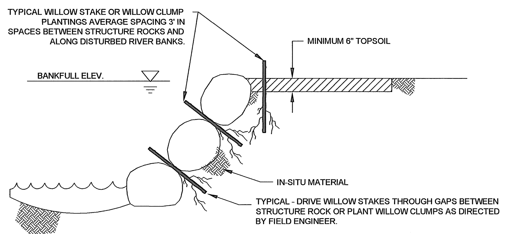
TYPICAL SECTION AT CROSS VANE (N.T.S.)
