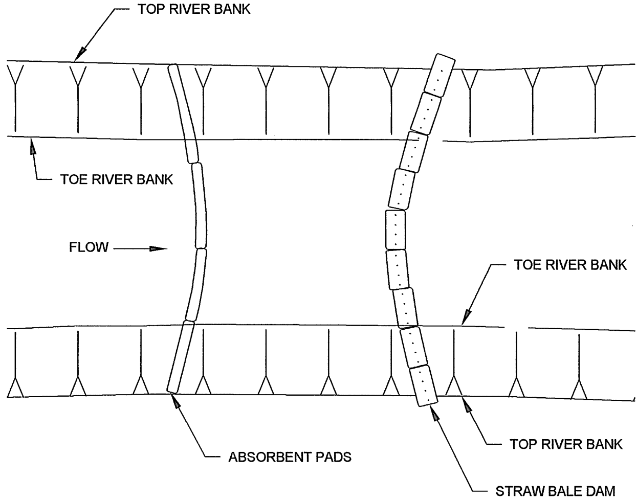
STRAW BALE DAM DETAIL (N.T.S.)
