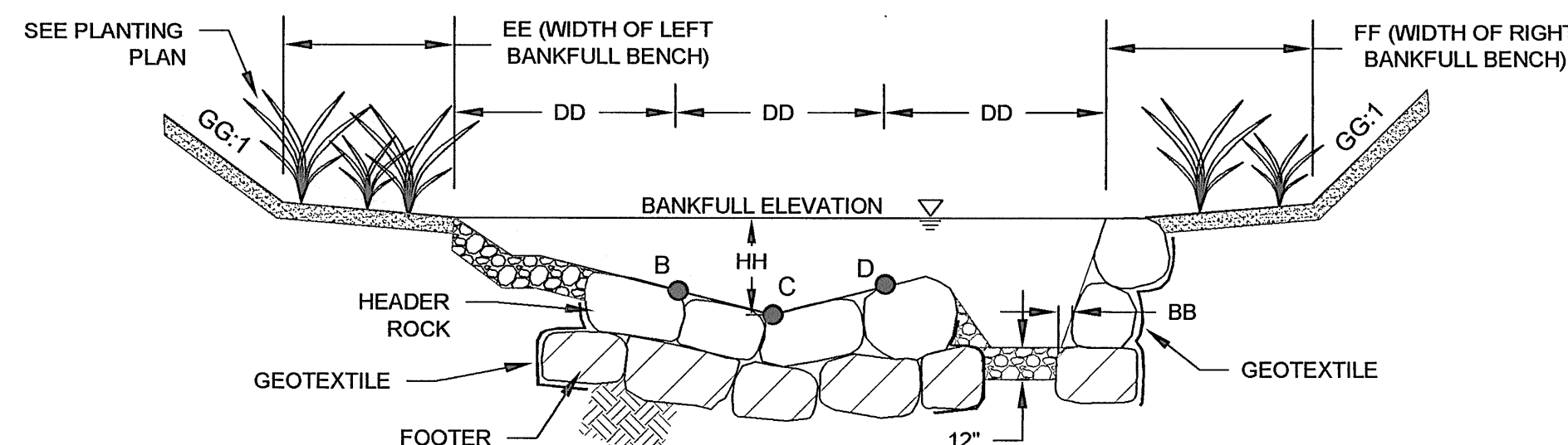
XS2 (N.T.S.)
