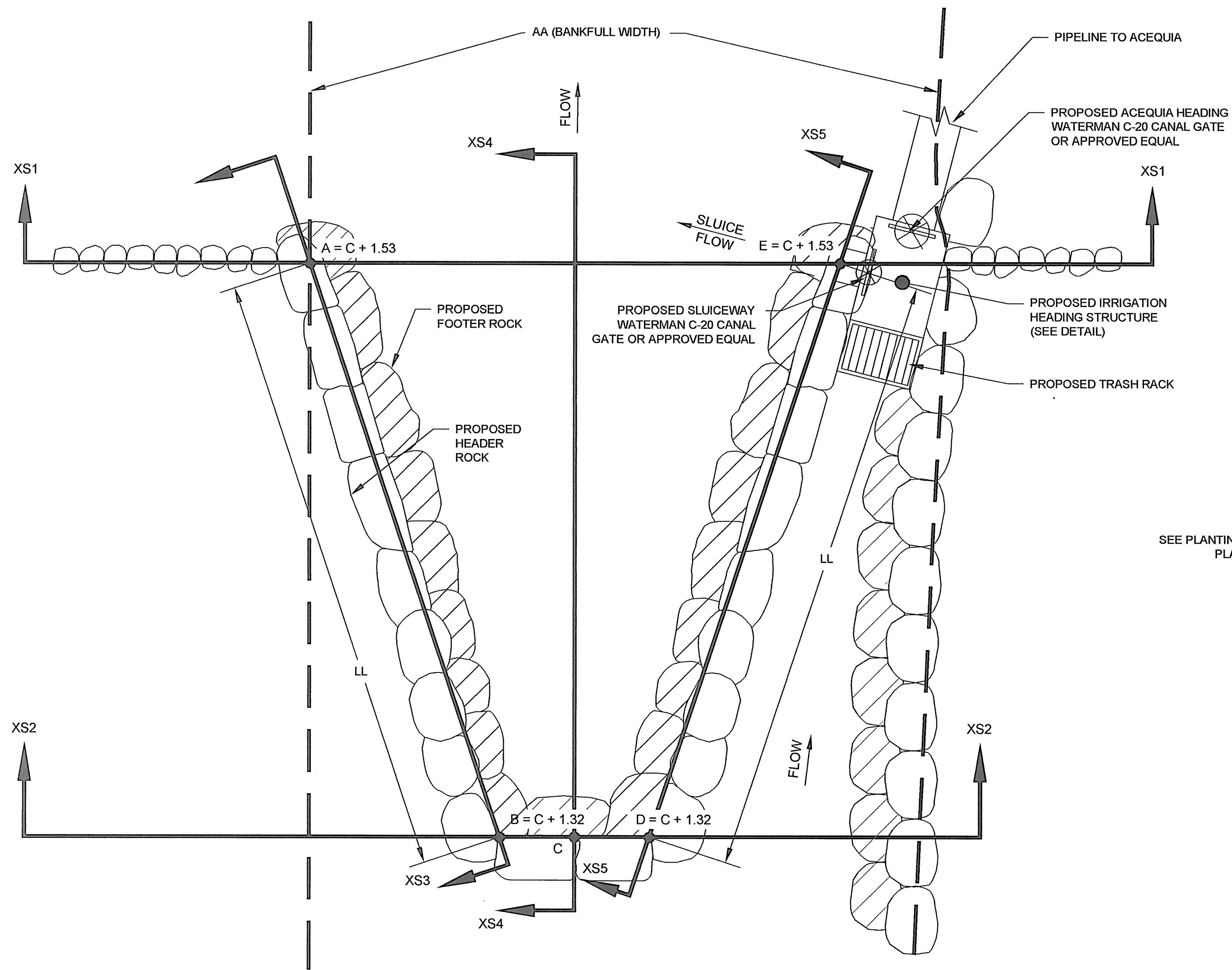
CROSS-VANE IRRIGATION HEADING STRUCTURE (N.T.S.)
