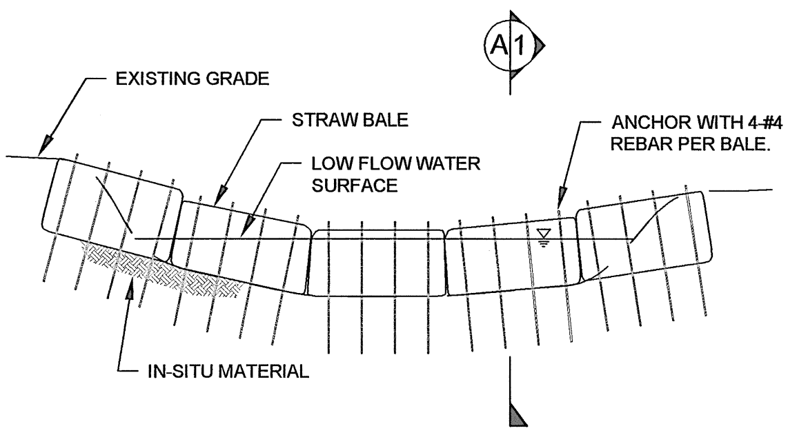
STRAW BALE DAM PLAN (N.T.S.)
